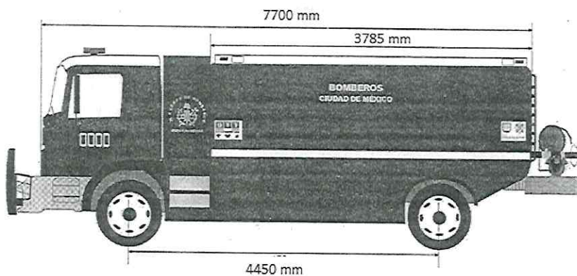
VISTA LATERAL
