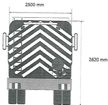
VISTA TRASERA
