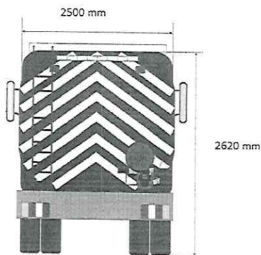
VISTA TRASERA
